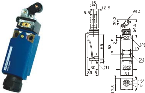
LL3XCPR2118P20 热塑滚轮摇杆
