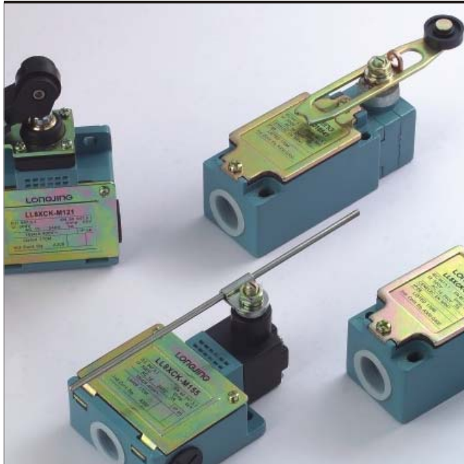
接触形式Contact Type 4回路双断型
